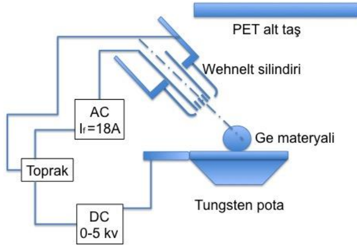
Şekil 1: TVA kaplama sisteminin şematik gösterimi
