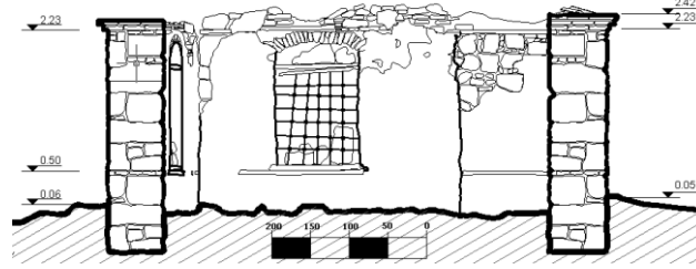
A-A KESİTİ (RÖLÖVE)
