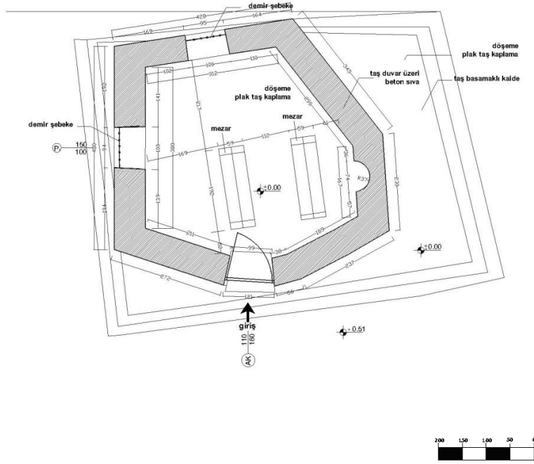
Plan şeması
