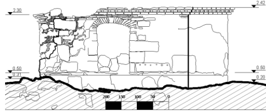
KUZEY CEPHESİ
