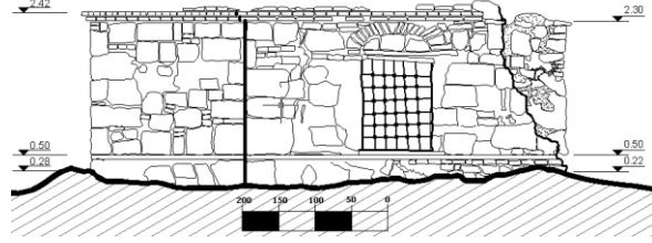
BATI CEPHESİ
