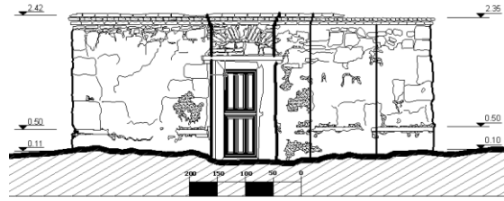
DOGU CEPHESİ
