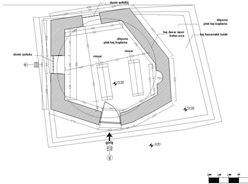
PLAN (RESTORASYON)
