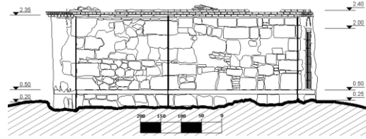
KUZEY CEPHESİ
