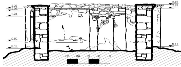
B-B KESİTİ (RÖLÖVE)
