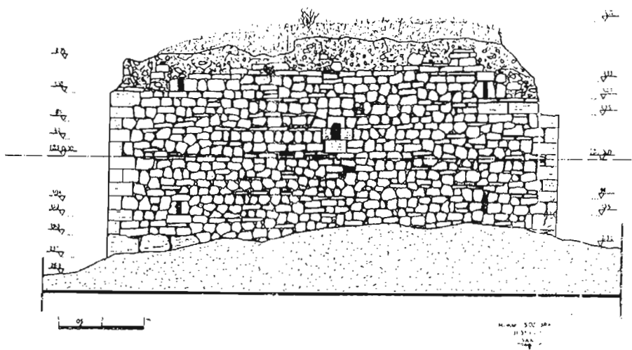
ÇİZİM-11: SURP VARDAN KİLİSESİ DOĞU CEPHE RÖLÖVESİ
