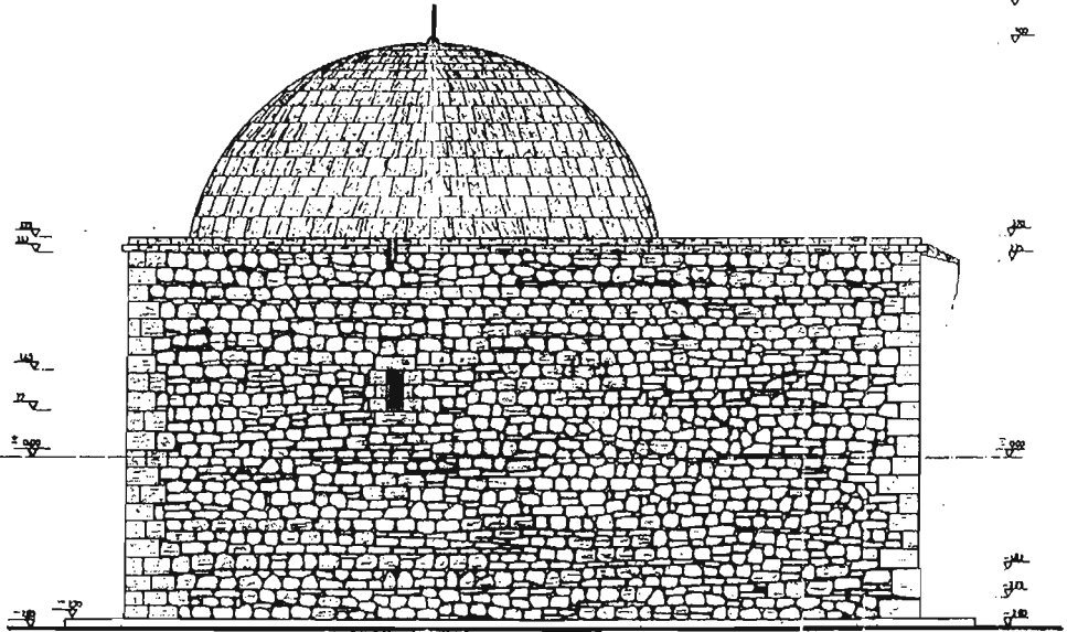
ÇİZİM-12: SURP VARDAN KİLİSESİ GÜNEY CEPHE RESTİTÜSYONU
