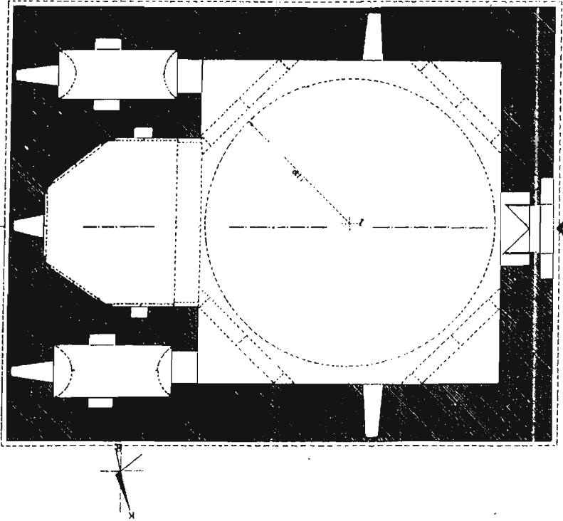
ÇİZİM-4: SURP YARDAN KİLİSESİ RESTİTÜSYON PLANI
