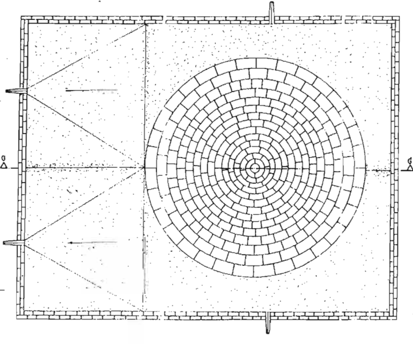
CİZİM-4 -SURP VARDAN KİLİSESİ ÖRTÜ SİSTEMİ RESTİTÜSYONU
