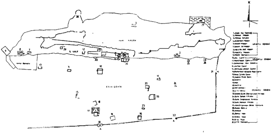
ÇİZİM-1 ESKİ VAN ŞEHİRİ VAZİYET PLANI
