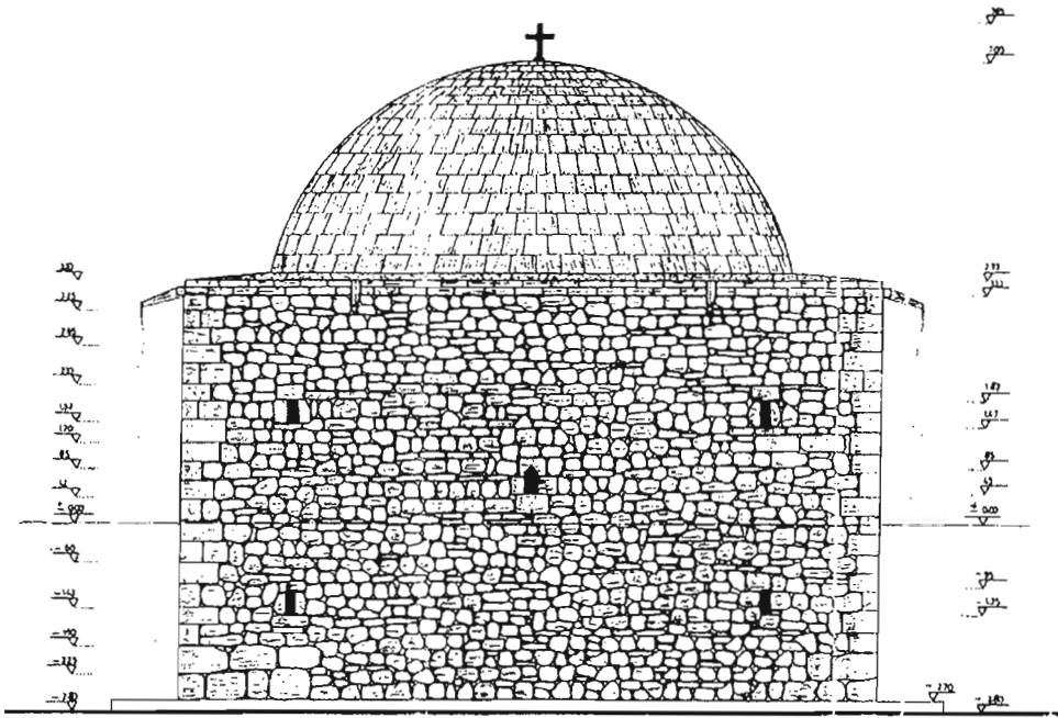
ÇİZİM-10: SURP VARDAN KİLİSESİ DOĞU CEPHE RESTİTÜSYONU
