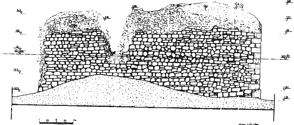
ÇİZİM-13: SURP VARDAN KİLİSESİ GÜNEY CEPHE RÖLİEFESİ
