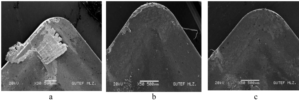
Şekil 4 Kesici uçların Scan Elektron Mikroskopi ile inlenmesinde oluşan aşınma ve BUE
