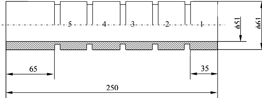
Şekil 1 Numunelerin Teknik Resmi
