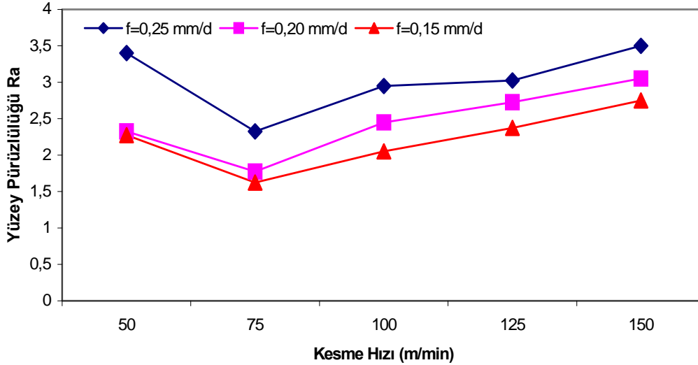
Şekil 5 İlerleme hızının yüzey pürüzlülüğüne etkisi
