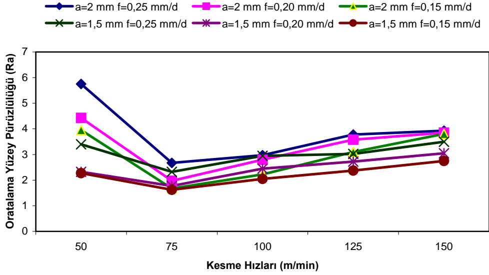
Şekil 3 Farklı kesme hızlarının, ilerlemenin ve talaş derinliğinin yüzey pürüzlülüğüne etkisi
