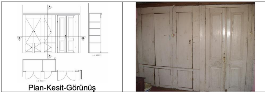
Şekil 5: 4 nolu yüklük
