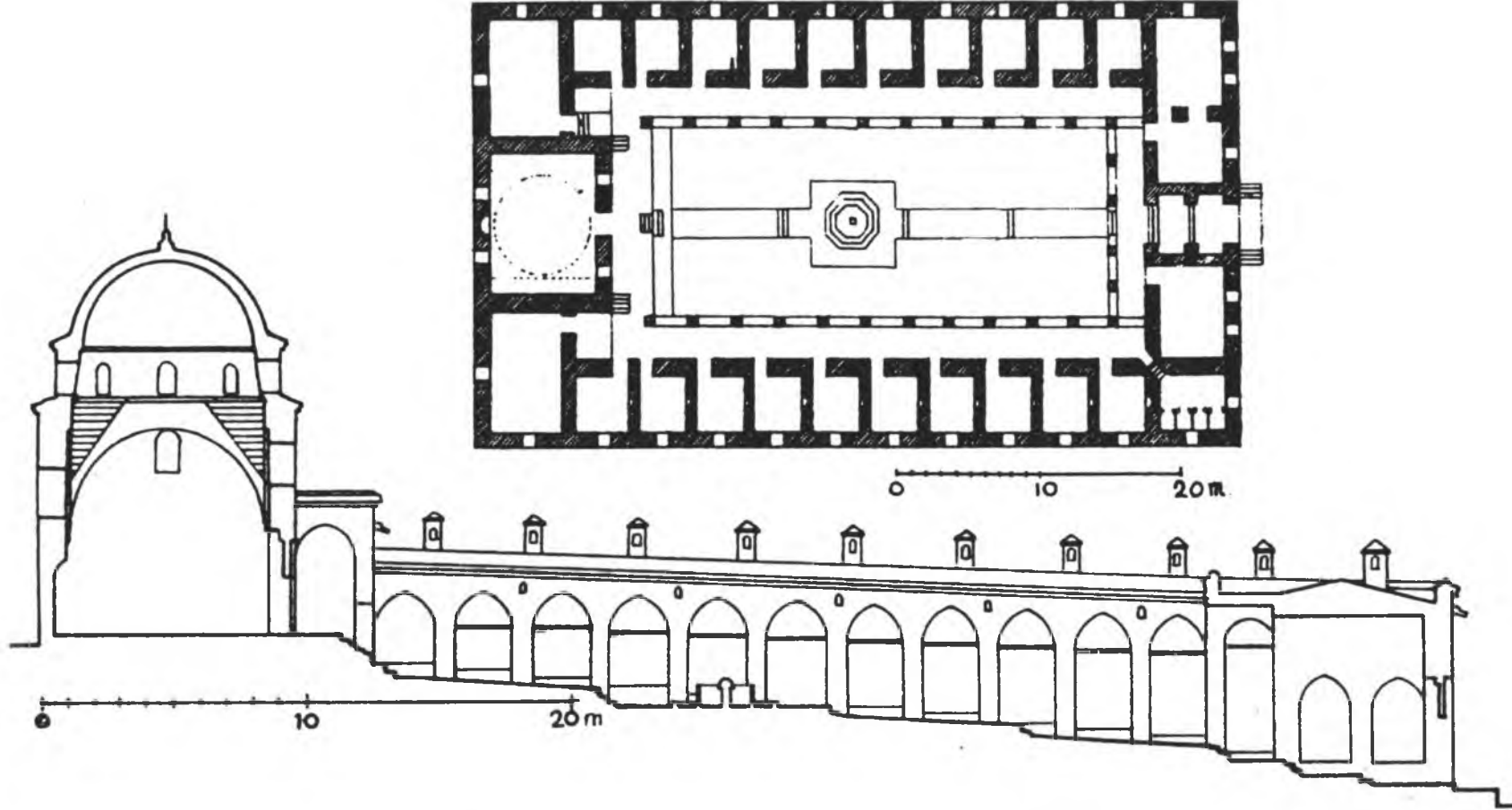
Pl. 3. Bursa, Yıldırım Külliyesi vaziyet plânı ve Darüşşifa plânı (A. Gabriel'den).
