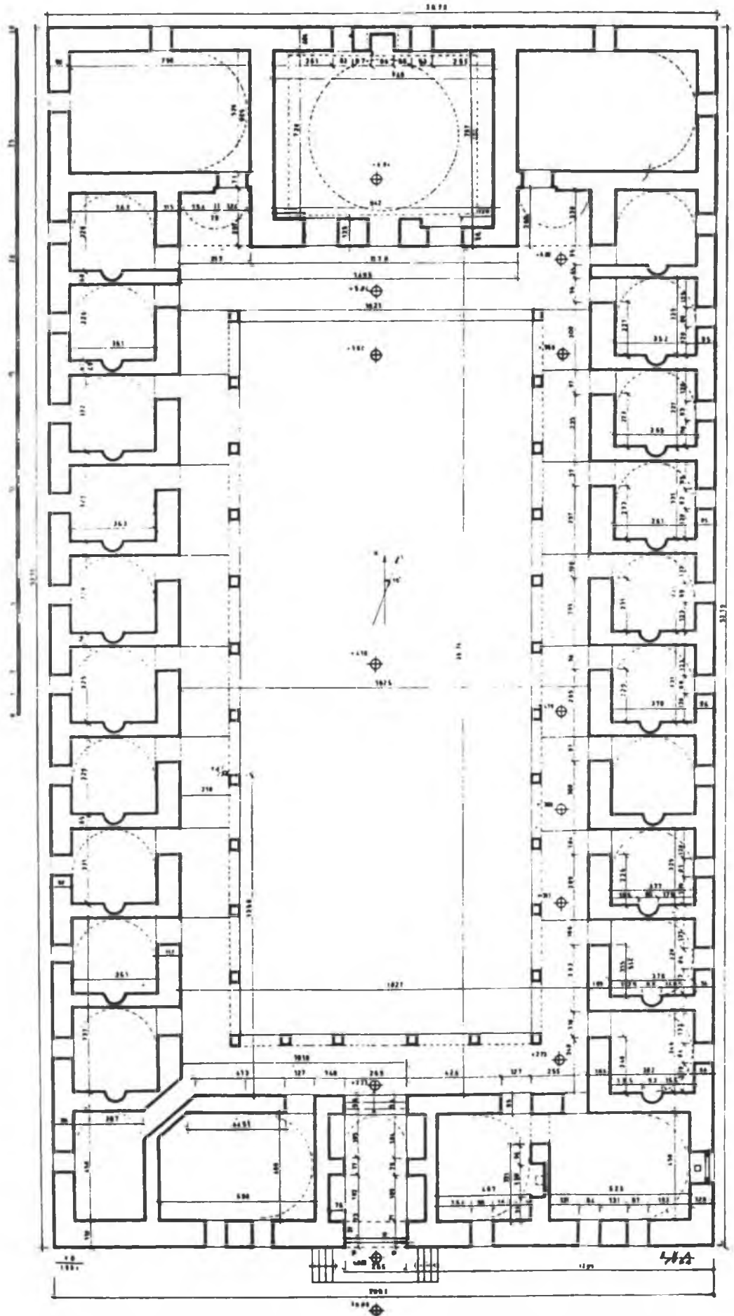
Pl. 4. Bursa, Yıldırım Külliyesi Darüşşifa plânı (E.H. Ayverdi'den).
