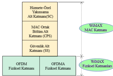
Şekil 3. Wimax MAC Katmanı ve OFDM-OFDMA Fiziksel Katmanı [17]
