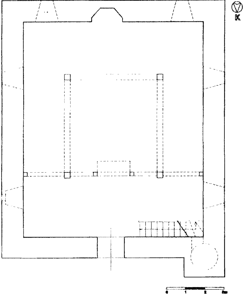
Erzurum / İlca- Alaca Köyü Camii Plan Rölövesi (03.10.2000)
