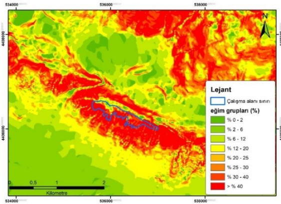
Şekil 2. Çalışma alanına ait eğim derecesi gruplarının dağılımı
