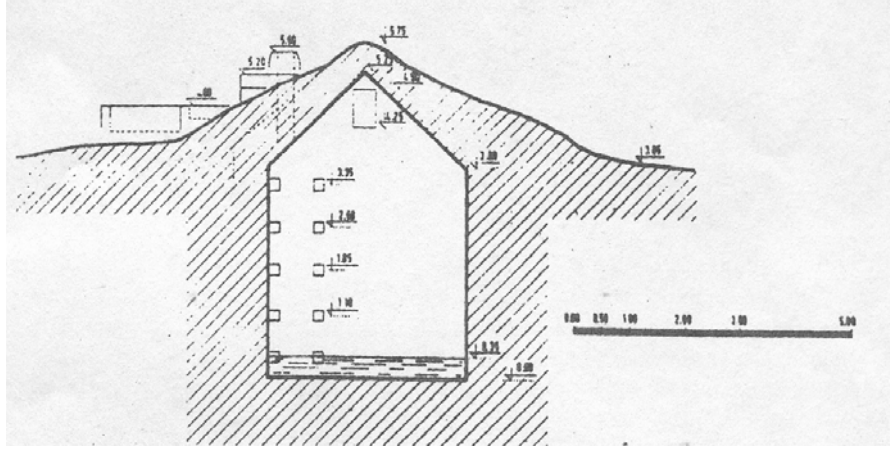
Buzlukbaşı Sarıncı Kesiti (H. Karpuz, Türk Kültür Varlıkları Envanteri'nden)
