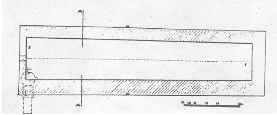
Buzlukbaşı Sarıncı Planı (Haşim Karpuz, Türk Kültür Varlıkları Envanteri'nden)
